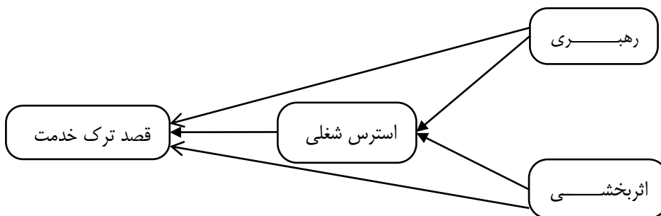
شکل ۱: مدل تحقیق
